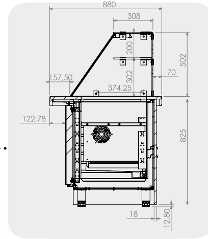
Ölçü Detayları Dimension Details
